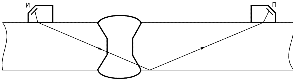
Рисунок 2. Зеркально-теневого
