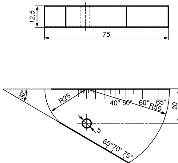
Рисунок Б.3. Эскиз НО V2
