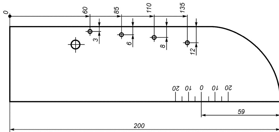
Рисунок А.3. Эскиз меры СО-3P
