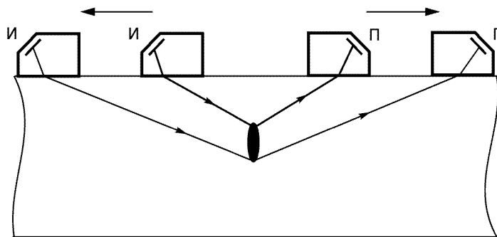
Рисунок 5. Дифракционный
