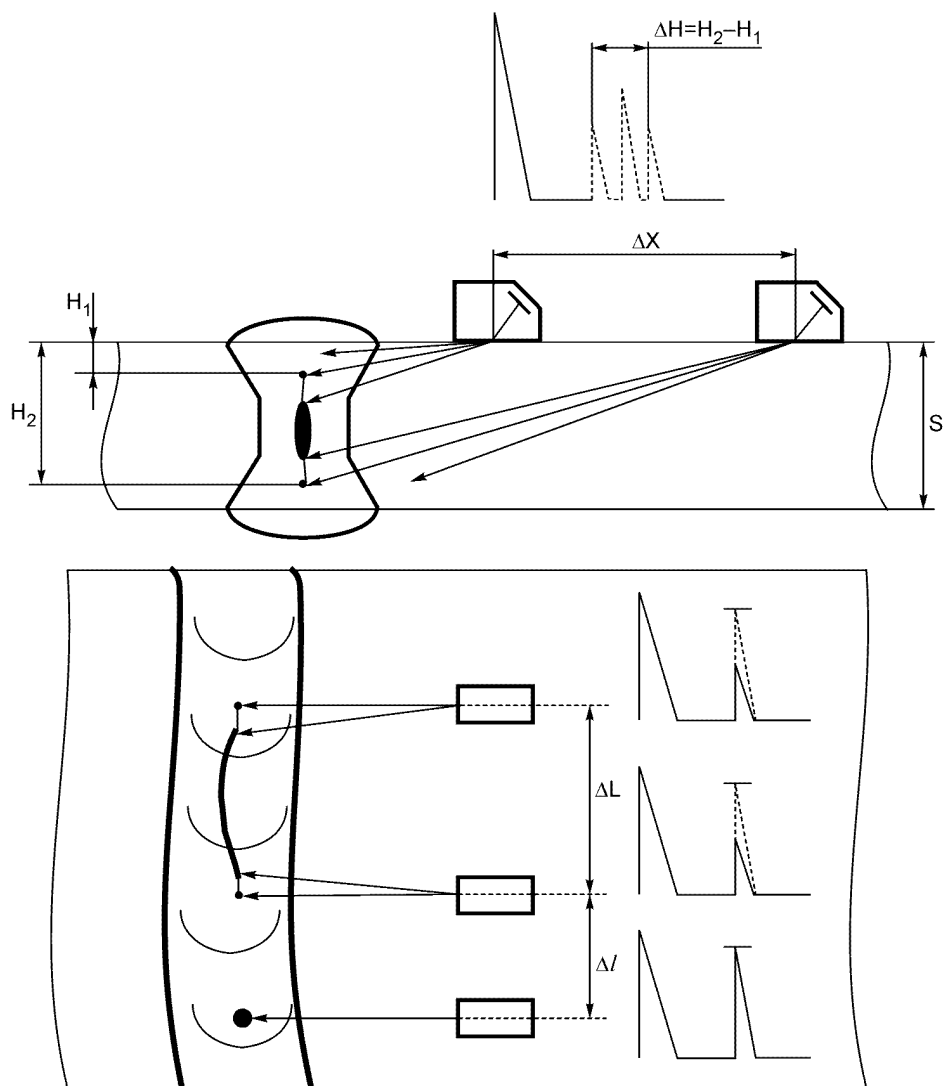
Рисунок 23. Измерение условных размеров дефектов
