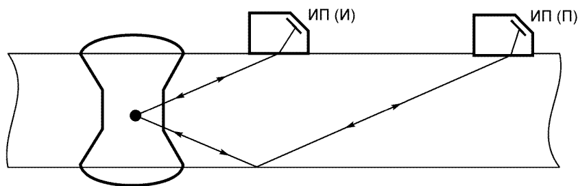
Рисунок 4. Эхо-зеркальный
