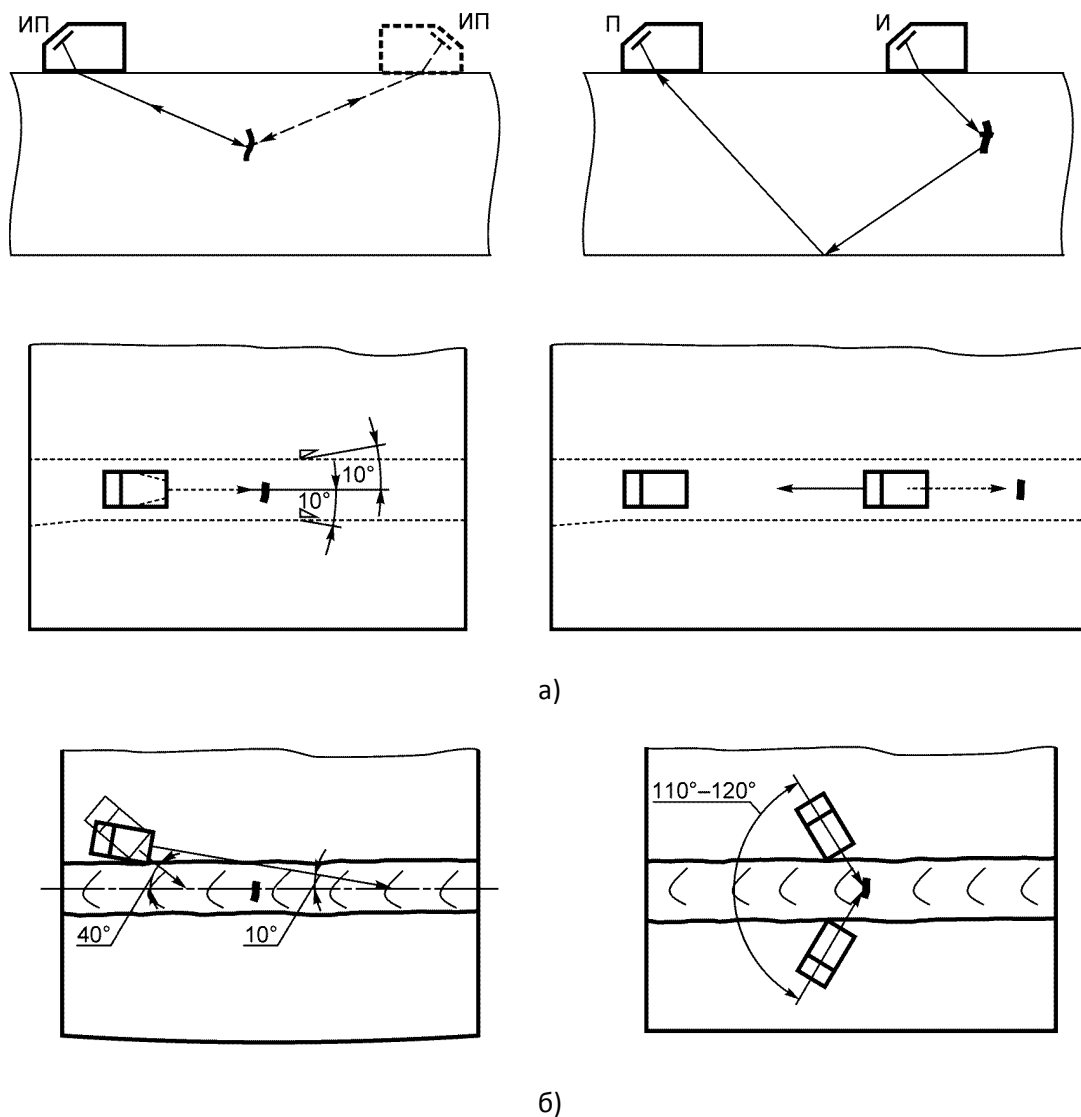
Рисунок 17. Схема прозвучивания стыковых сварных соединений при контроле для поиска поперечных трещин: а) - со снятым валиком шва; б) - с неудаленным валиком шва
