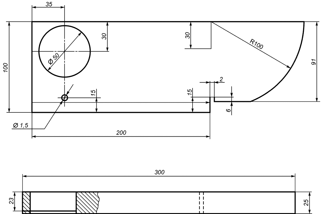
Рисунок Б.2. Эскиз НО V1
