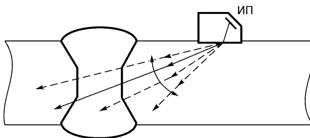
Рисунок 21. Способ сканирования качающимся лучом
